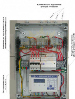
Демонстрационный стенд по электроснабжению (крышка снята).
