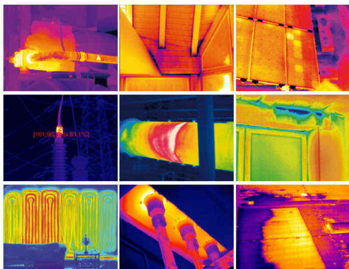
Рис. 3. Примеры термограмм с тепловизором Trotec
