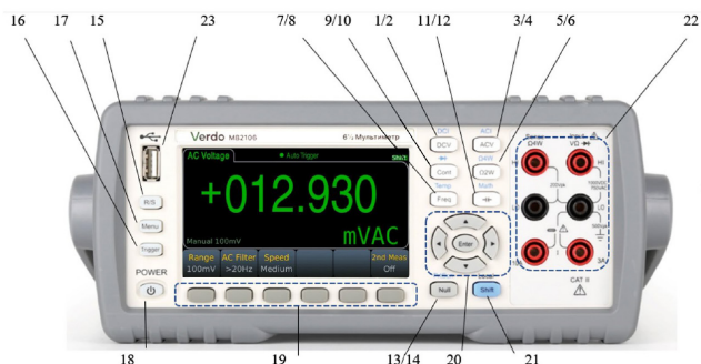
Передняя панель VERDO MB2105/2106/2107
