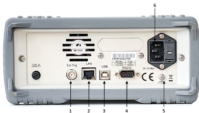
Задняя панель VERDO MB2106
