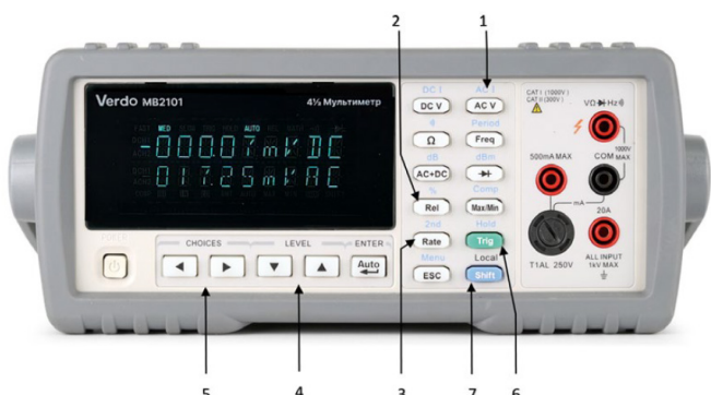
Передняя панель VERDO MB2101 и MB2102
