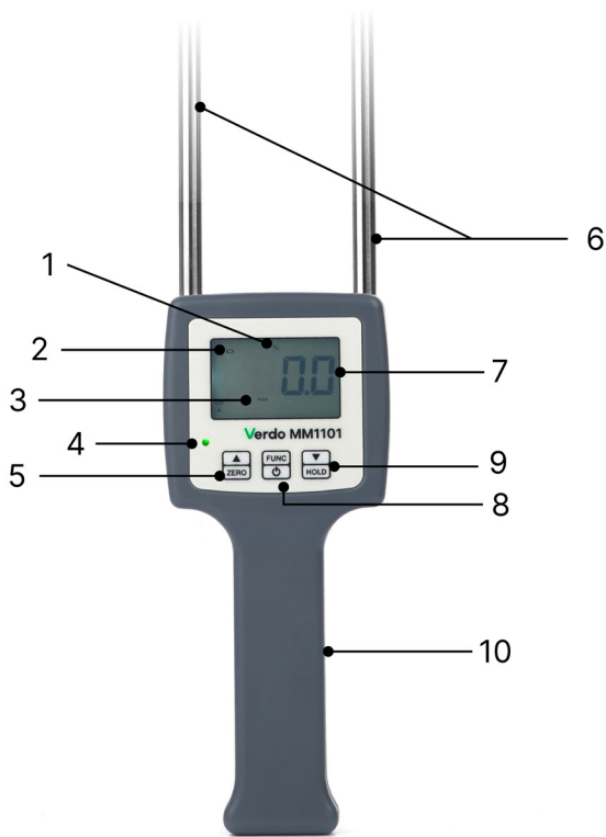
Рисунок 1 – Внешний вид влагомера
