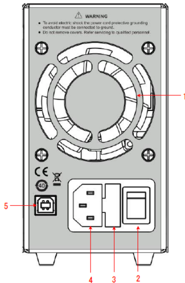
Рисунок 2-3 Обзор задней панели
