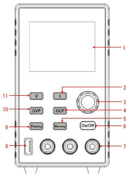
Рисунок 2-2 Передняя панель
