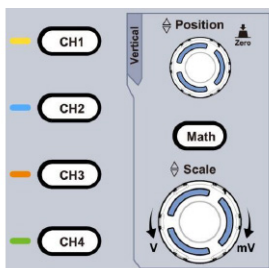
Рисунок 9 - Зона управления вертикальной разверткой
