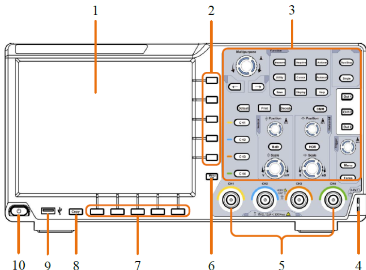
Рисунок 1 - Передняя панель
