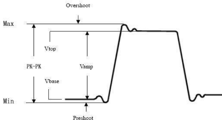
Рисунок 30 - Импульс с некоторыми точками измерения напряжения
