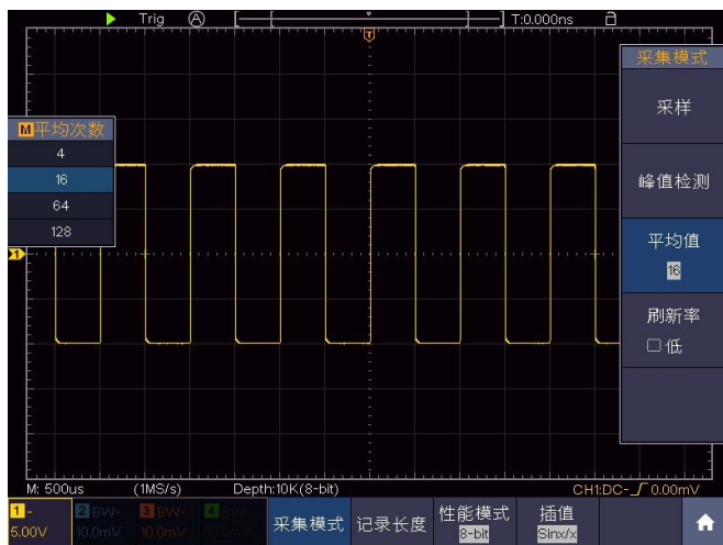
Рисунок 53 - Снижение уровня шума с помощью функции усреднения
