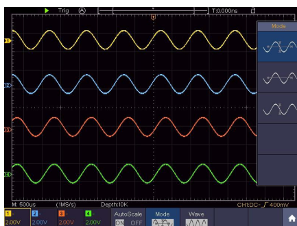
Рисунок 34 - Горизонтально-вертикальное автоматическое масштабирование многопериодных сигналов
