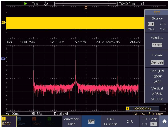
Рисунок 16 - Окно Кайзера
