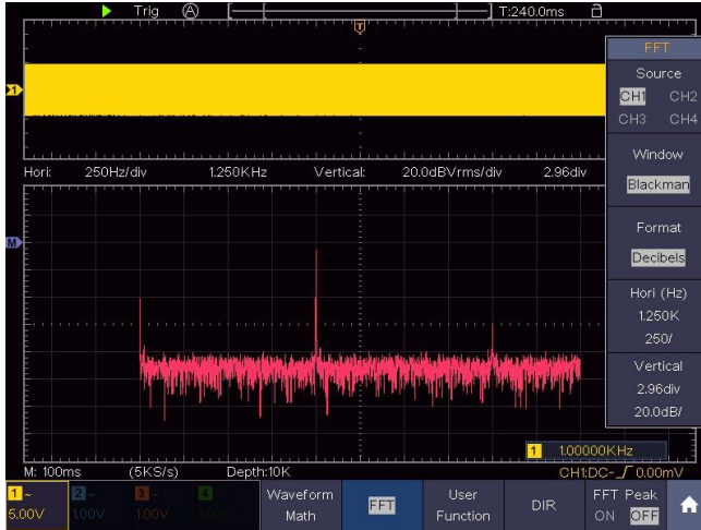
Рисунок 14 - Окно Блэкмена
