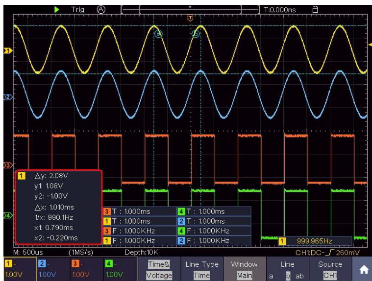
Рисунок 32 - Измерение времени и напряжения курсора
