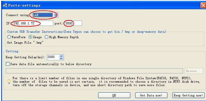
Рисунок 47 - Установка сетевых параметров осциллографа
