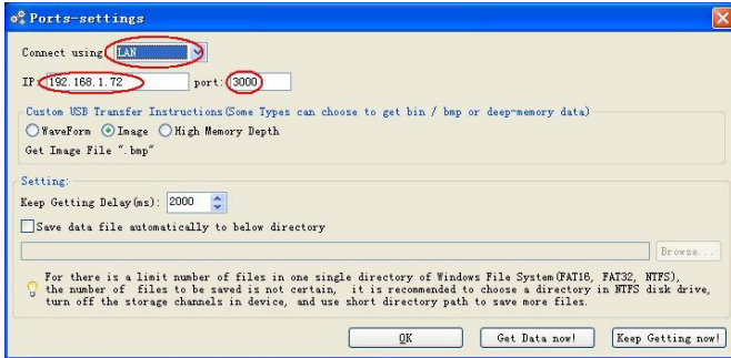
Рисунок 44 - Настройка сетевых параметров программного обеспечения осциллографа
