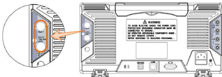
Рисунок 35 - Выходные порты генератора (двухканальные)
