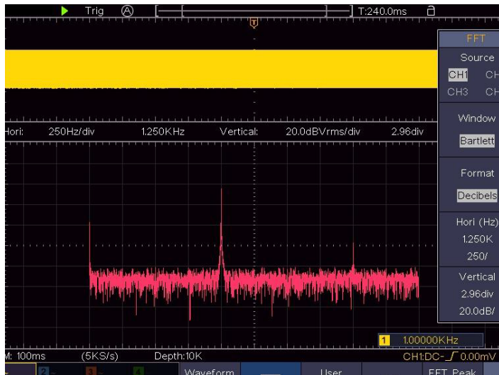
Рисунок 17 - Окно Бартлетта
