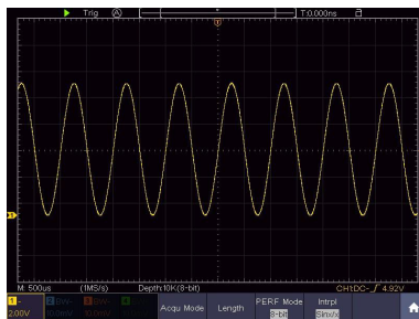
Рисунок 21 - интерполяция \sin(x)/x
