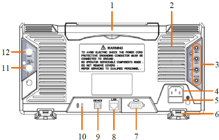
Рисунок 2 - Задняя панель
