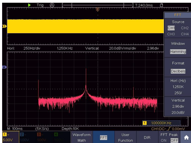
Рисунок 12 - Окно Хэмминга
