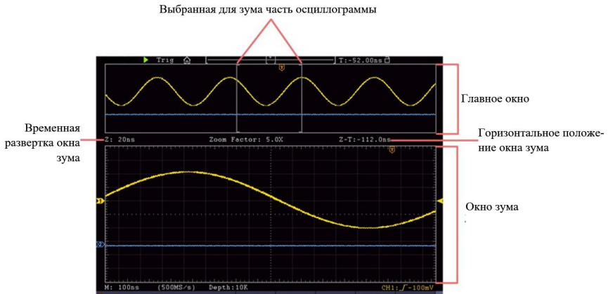
Рисунок 19 - Режим горизонтального масштабирования осциллограммы
