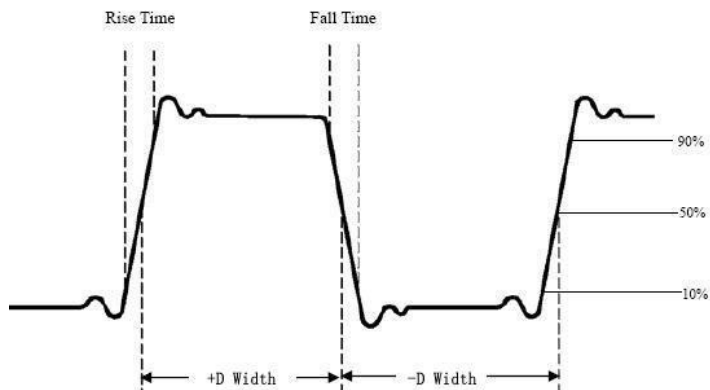
Рисунок 31 - Импульс с некоторыми точками измерения времени
