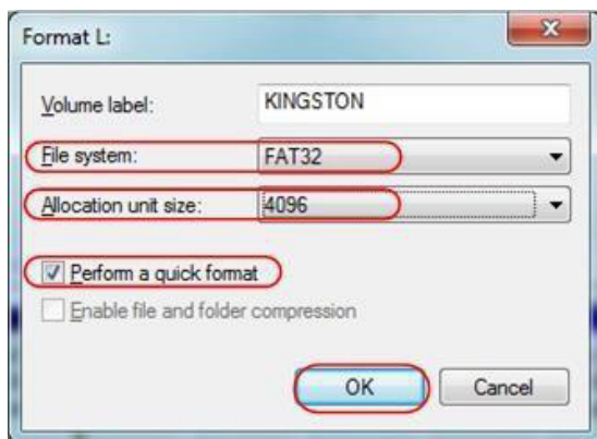
Рисунок 26 - Форматирование USB-диска
