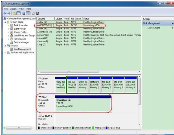
Рисунок 27 - Форматирование USB-диска
